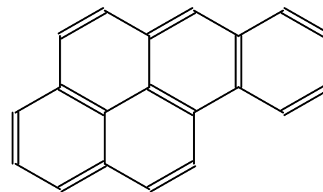
۱ و ۲ بنزپیرن
