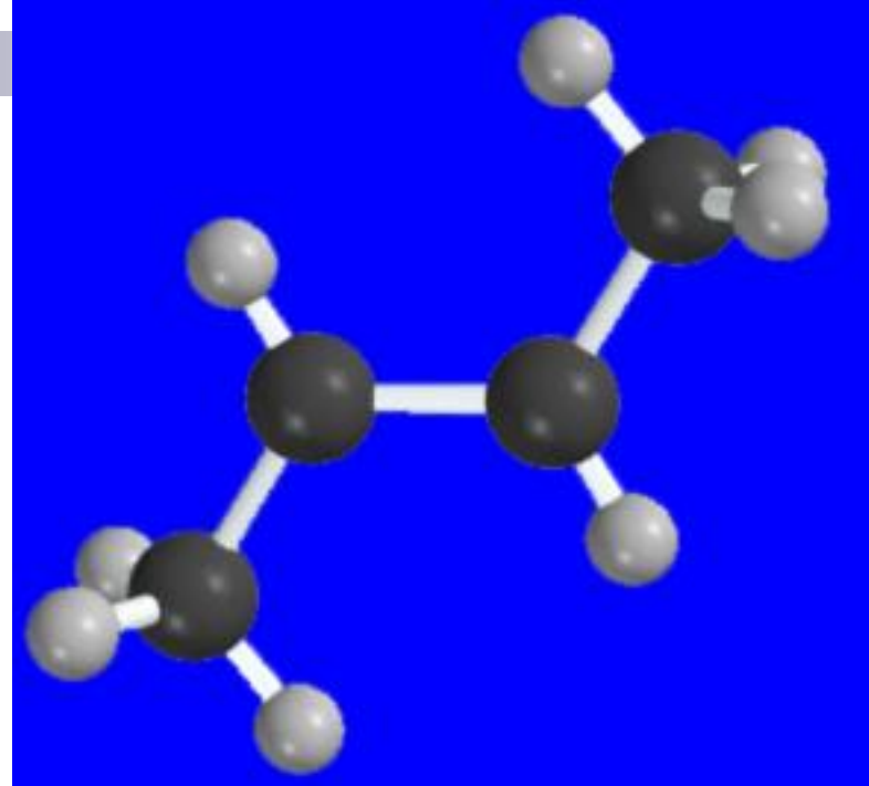
ترانس ۲ - بوتن
