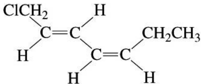
(2E,4Z)-1-chloro-2,4-heptadiene
