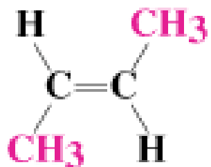
trans-2-Butene
